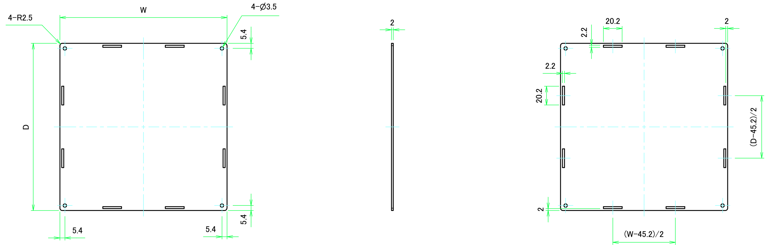
上カバー裏面 / Top cover Backside
